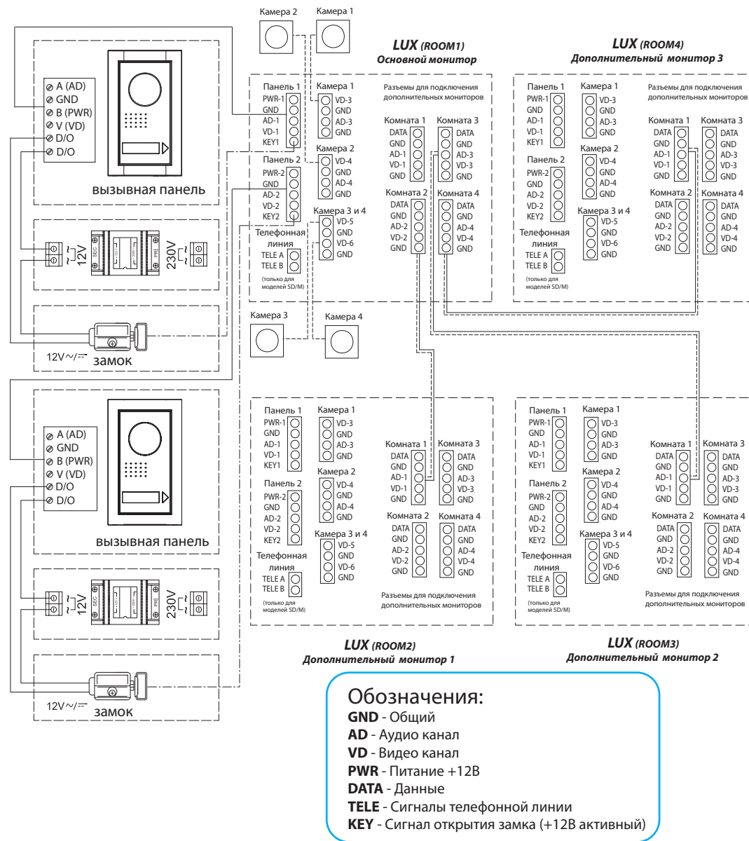
Рис. 1. Схема подключения двух вызывных панелей, четырех видеокамер и двух замков к системе видеодомофонов GARDI LUX.
